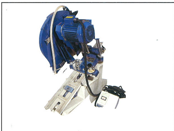
Dispositivo per il taglio di gradini applicabile a tutte le taglie-muri
