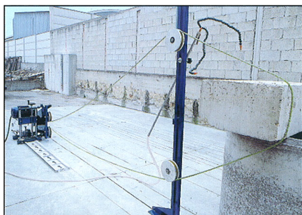
Taglio a filo a senso verticale mediante l'ausilio del telaio mobile con estremità regolabile per fissarla al soffitto e fissandola sul pavimento (in dotazione)
