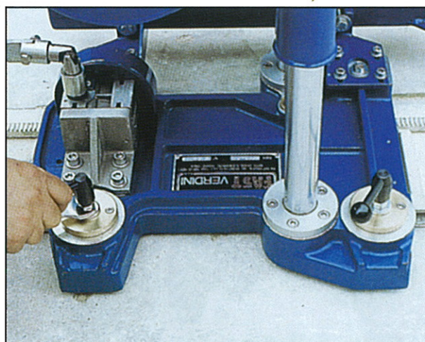
Nuovo sistema di fissaggio delle due carrucole su binari a eccentrico che evita qualsiasi gioco.
