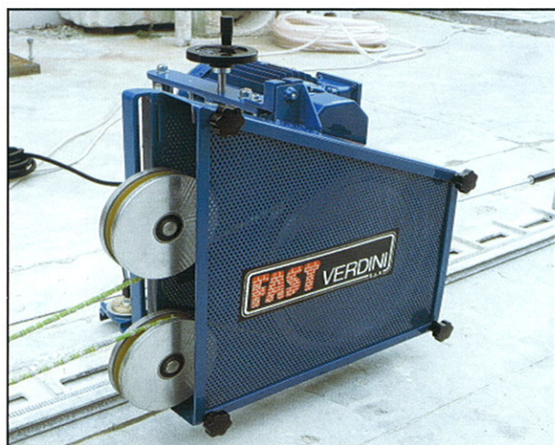
Testata del comando filo diamantato.
